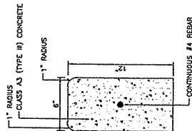
TYPE 7 P.C.C. PARK CURB
